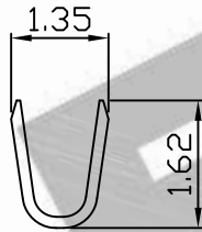
SEC A-A
